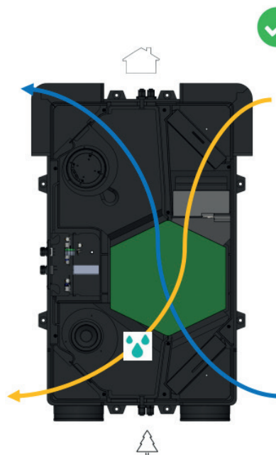
Montaż z przełącznikiem ustawionym w pozycji „lewej”
